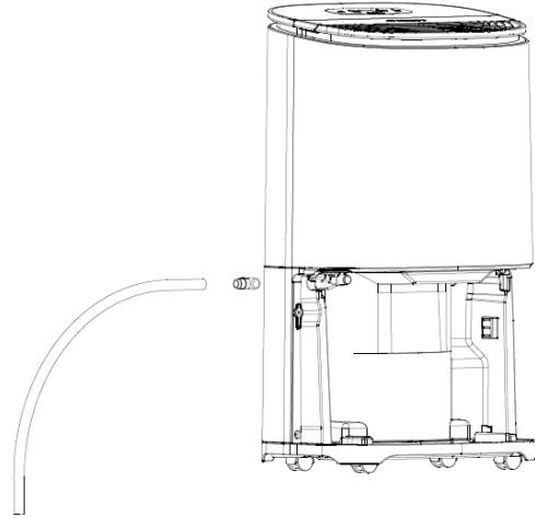
Vaihe 2: Irrota oikean kulman sovitin vesisäiliön kannesta ja työnnä se nokan päälle. Nokka on siinä kohdassa, josta vesi tippuu kosteudenpoistajasta ja sijaitsee vasemmalla puolella.
